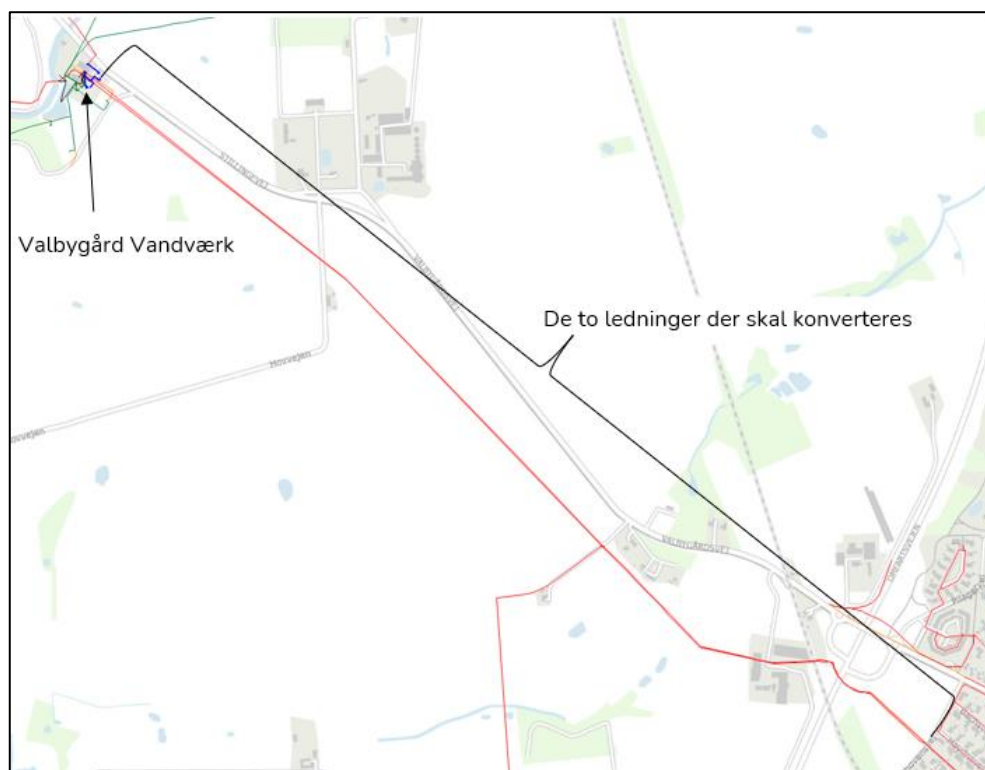
Figur 3. Rentvandsledninger som konverteres til råvandsledninger.
